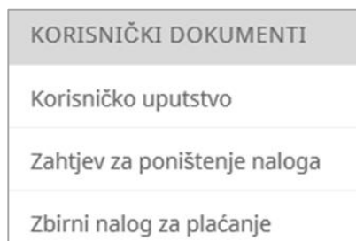
Slika 81: Korisnički dokumenti
