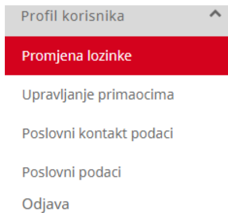
Slika 13: Profil korisnika
